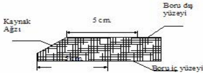
Şekil 12 Boru kaynak ağızı
